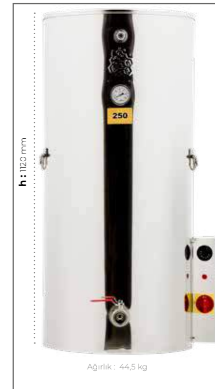
BA580-304 250 Kg Ø : 510 mm
